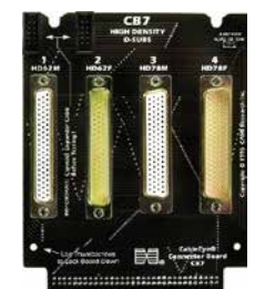
CB7 HD62, HD78 (Item 737)
